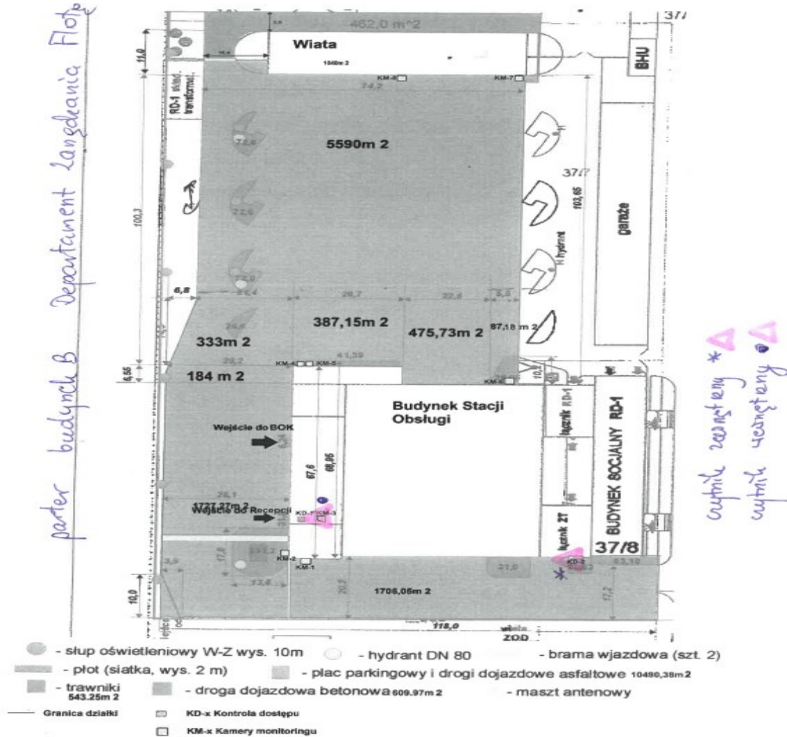
Plan sytuacyjny budynku i działki DZF
