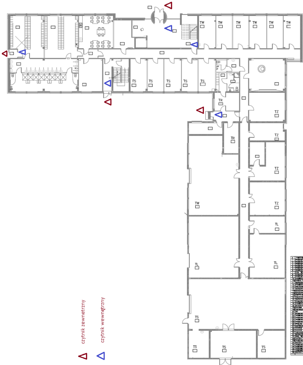
RZUT PARTERU
